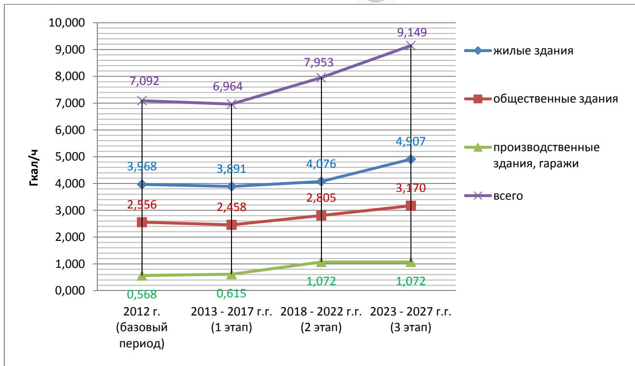
Рис. 1.11. Динамика изменения тепловых нагрузок в период до 2028 года
