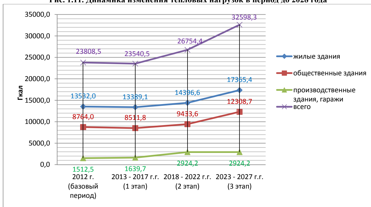
Рис. 1.12. Динамика изменения теплопотребления в период до 2028 года
